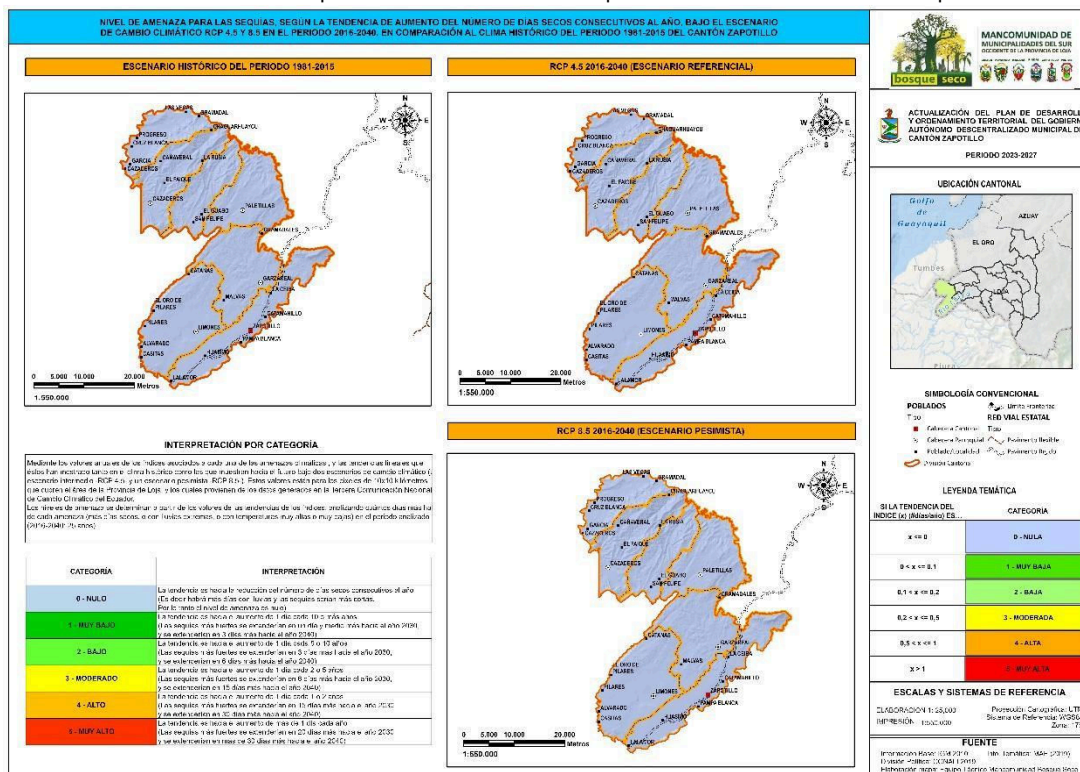
Mapa 14. Nivel de amenaza para las sequías, según la tendencia de aumento del número de días secos consecutivos al año, bajo los escenarios de cambio climático RCP 4.5 y RCP 8.5 en el periodo 2016-2040, en comparación al clima histórico del periodo 1981-2015 en el cantón Zapotillo
