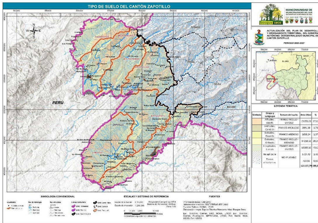
Mapa 5. Edafología en el cantón Zapotillo
