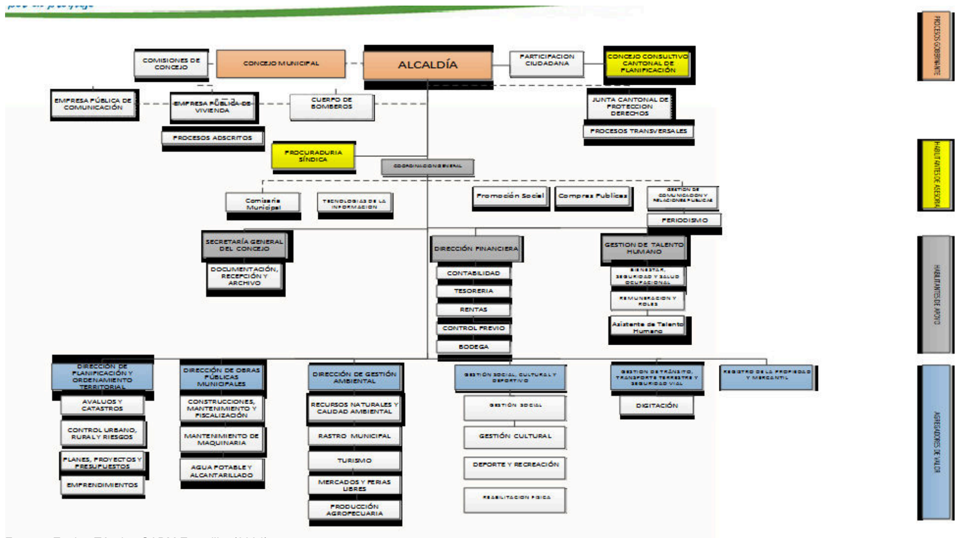
Figura 37. Organigrama estructural
