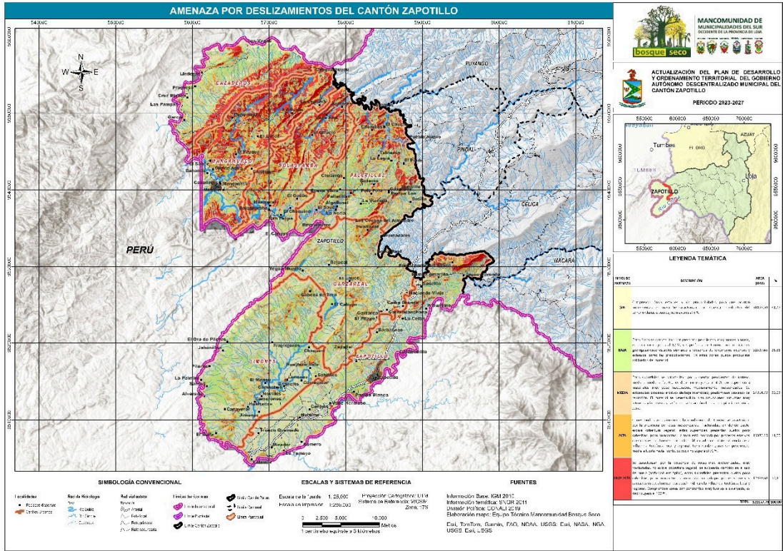
Mapa 11. Amenazas por deslizamientos en el cantón Zapotillo
