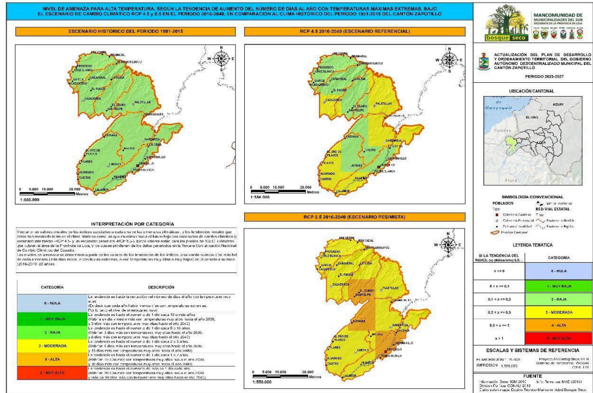
Mapa 16. Nivel de amenaza para alta temperatura, según la tendencia de aumento del número de días al año con temperaturas máximas extremas, bajo los escenarios de cambio climático RCP 4.5 y RCP 8.5 en el periodo 2016-2040, en comparación al clima histórico del periodo 1981-2015 en el cantón Zapotillo
