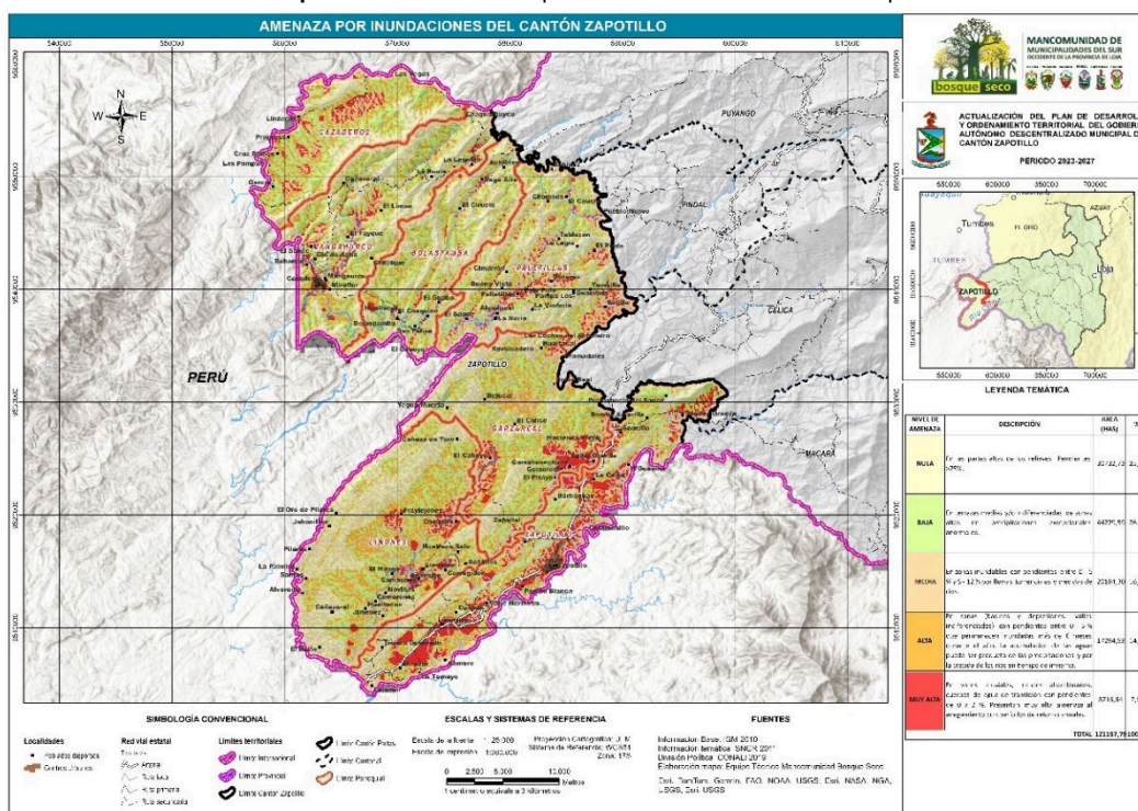
Mapa 12. Amenazas por inundaciones en el cantón Zapotillo
