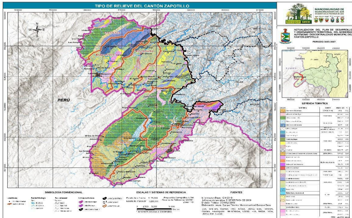
Mapa 4. Unidades geomorfológicas del cantón Zapotillo
