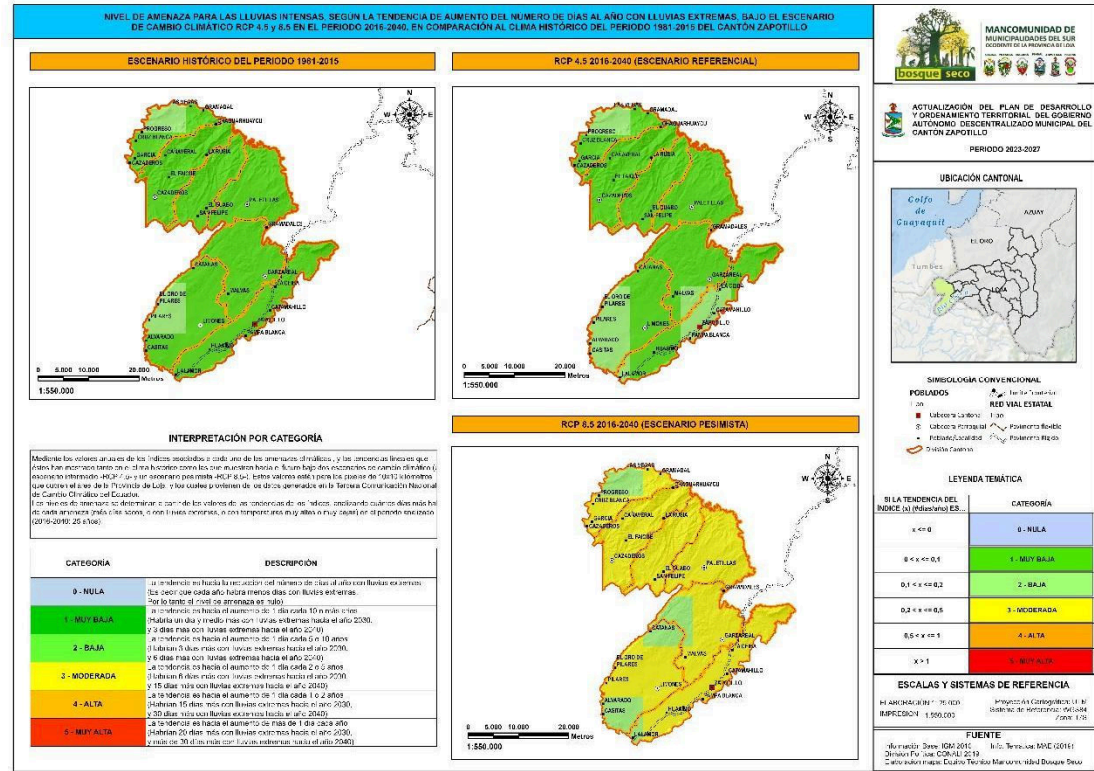
Mapa 15. Nivel de amenaza para las lluvias intensas, según la tendencia de aumento del número de días al año con lluvias extremas, bajo los escenarios de cambio climático RCP 4.5 y RCP 8.5 en el periodo 2016-2040, en comparación al clima histórico del periodo 1981-2015 en el cantón Zapotillo
