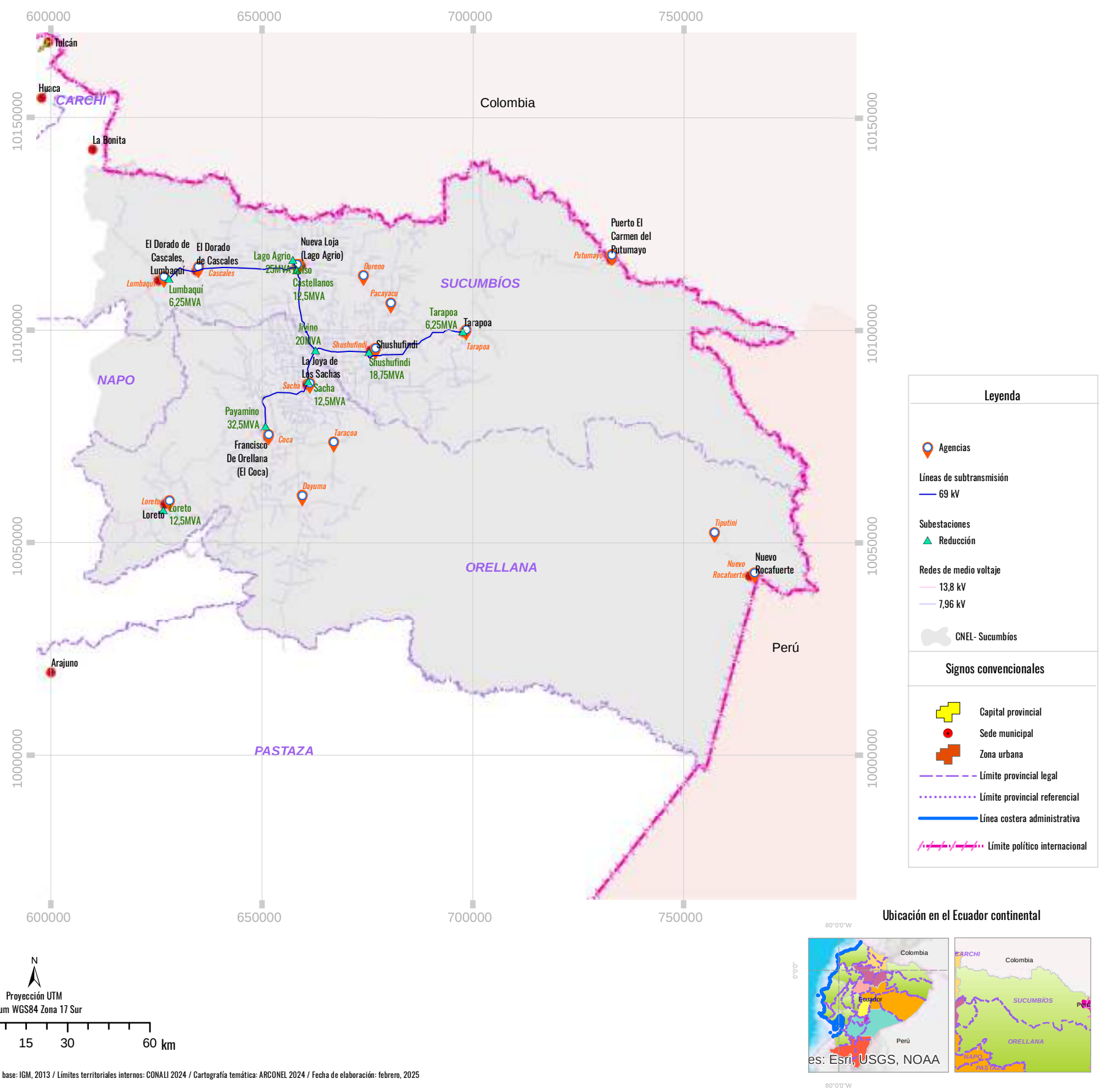
Mapa Nro 24: Infraestructura eléctrica de CNEL EP Unidad de Negocio Sucumbíos
