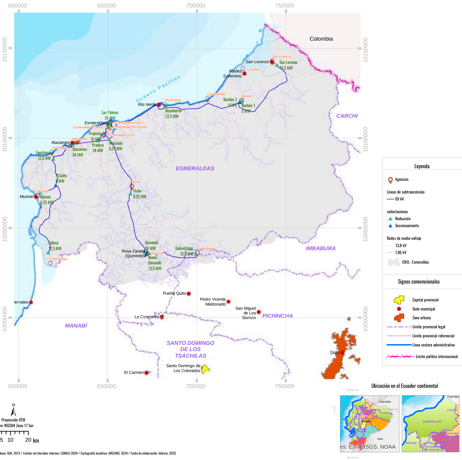
Mapa Nro. 16: Infraestructura eléctrica de CNEL EP Unidad de Negocio Esmeraldas
