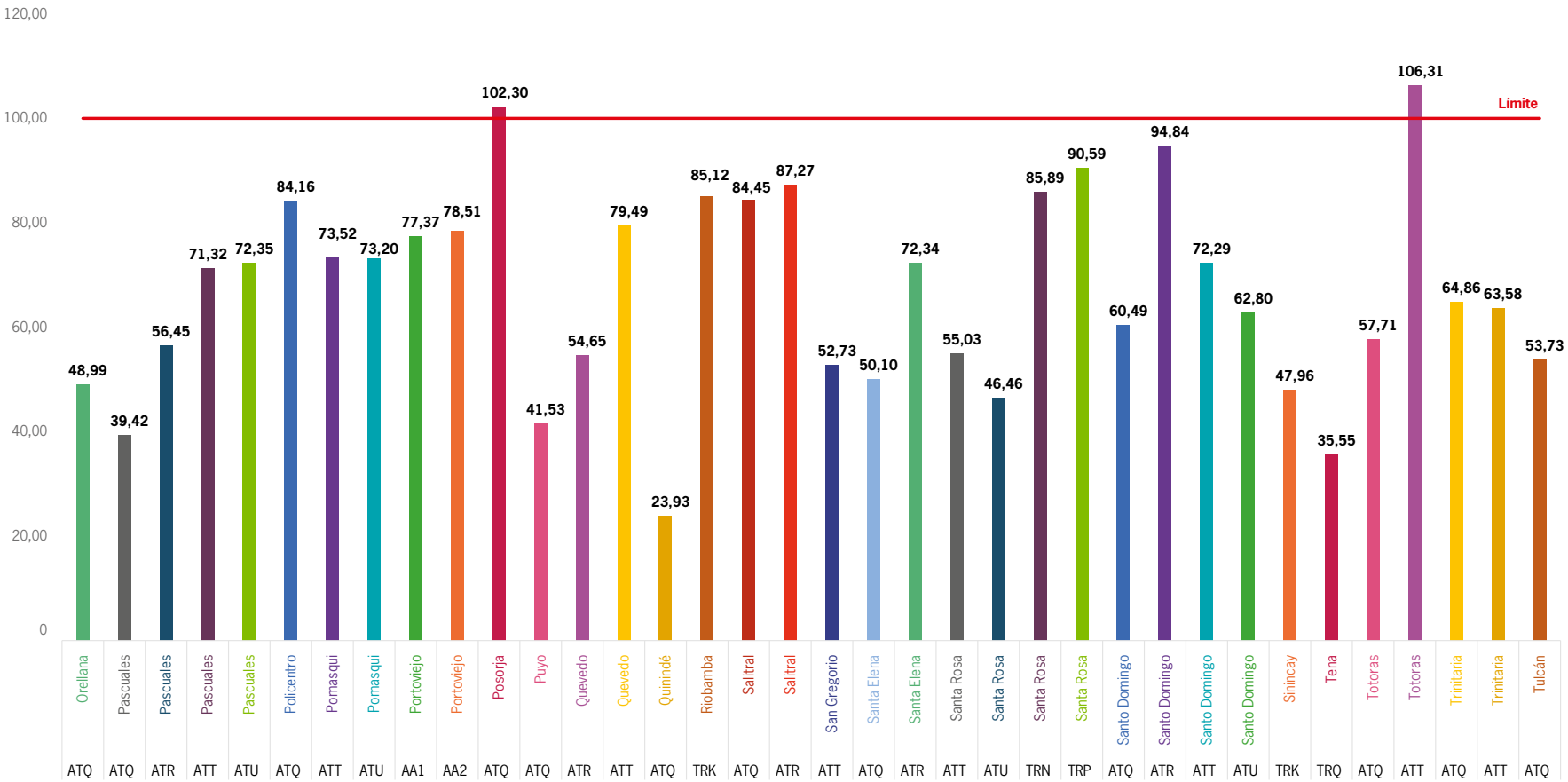
FIG. No. 51: CARGABILIDAD MÁXIMA DE TRANSFORMADORES DEL SNT (2/2)
