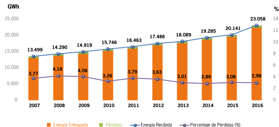
FIG. No. 118: PÉRDIDAS DE ENERGÍA EN EL SNT
