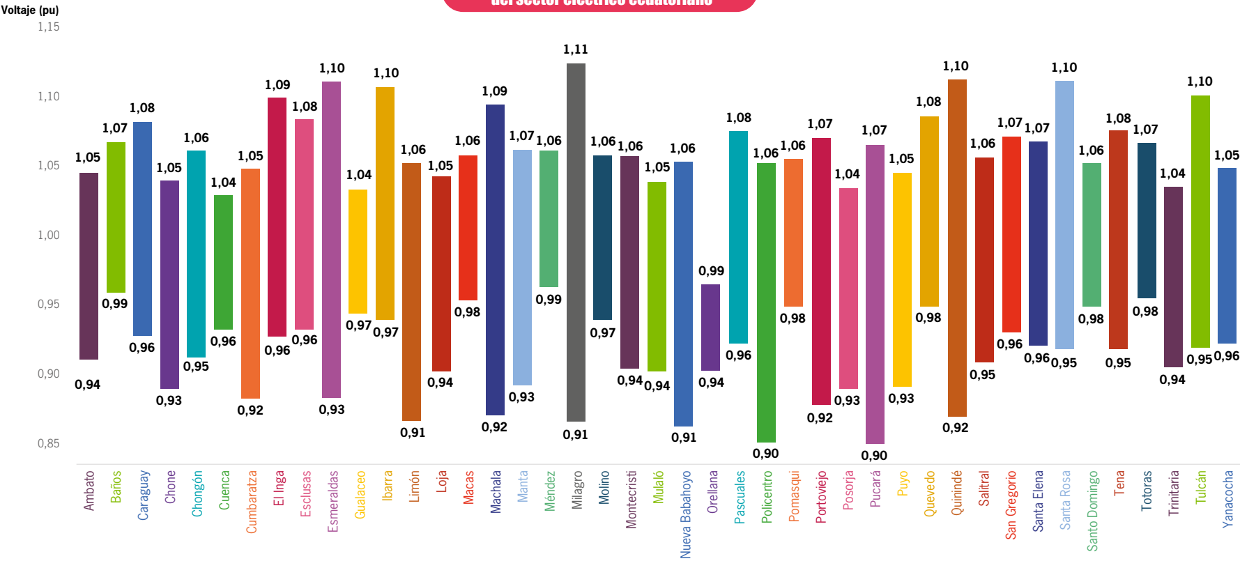
FIG. No. 50: VOLTAJES EN SUBESTACIONES DE 138 kV (pu)
