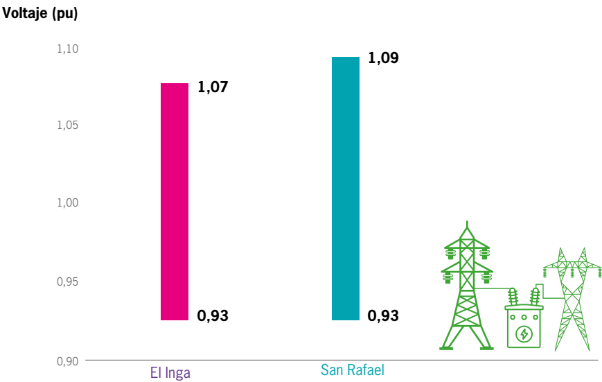
FIG. No. 48: VOLTAJES EN SUBESTACIONES DE 500 kV (pu)
