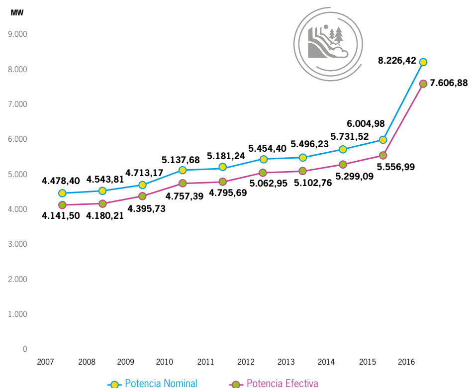
FIG. No. 104: EVOLUCIÓN HISTÓRICA DE LAS POTENCIAS NOMINAL Y EFECTIVA
