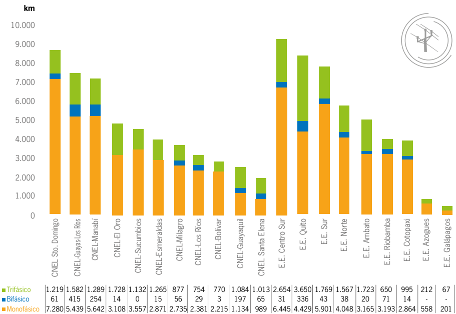
FIG. No. 15: LONGITUD DE REDES DE MEDIO VOLTAGE POR EMPRESA
