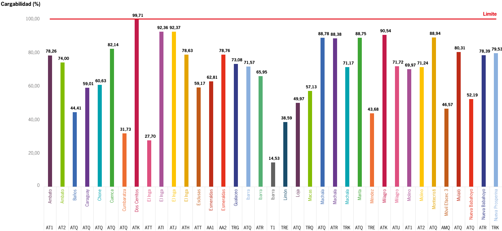
FIG. No. 51: CARGABILIDAD MÁXIMA DE TRANSFORMADORES DEL SNT (1/2)
