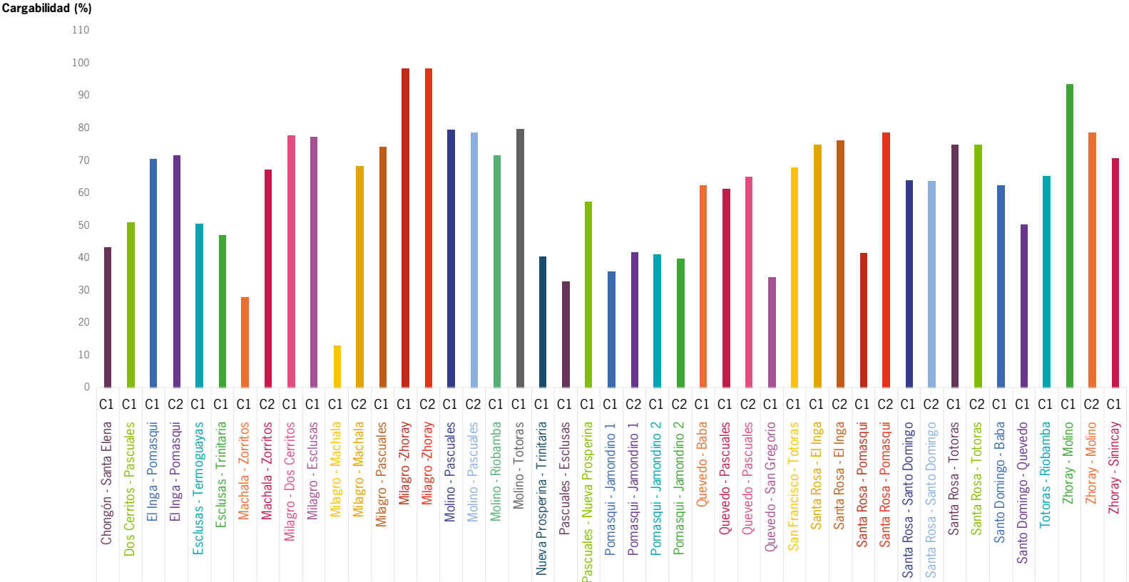
FIG. No. 53: CARGABILIDAD DE LÍNEAS DE 230 kV
