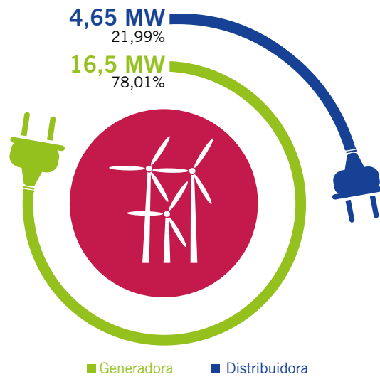
FIG. No. 6: POTENCIA EFECTIVA DE CENTRALES EÓLICAS POR TIPO DE EMPRESA
