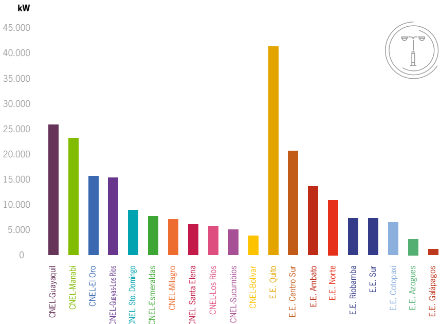
FIG. No. 18: POTENCIA INSTALADA DE LUMINARIAS (kW)
