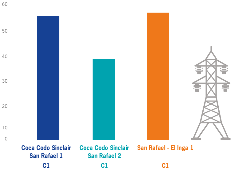
FIG. No. 52: CARGABILIDAD DE LÍNEAS DE 500 kV
